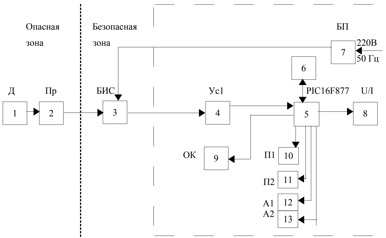
Рис.1. Структурная схема устройства ИП-107.
