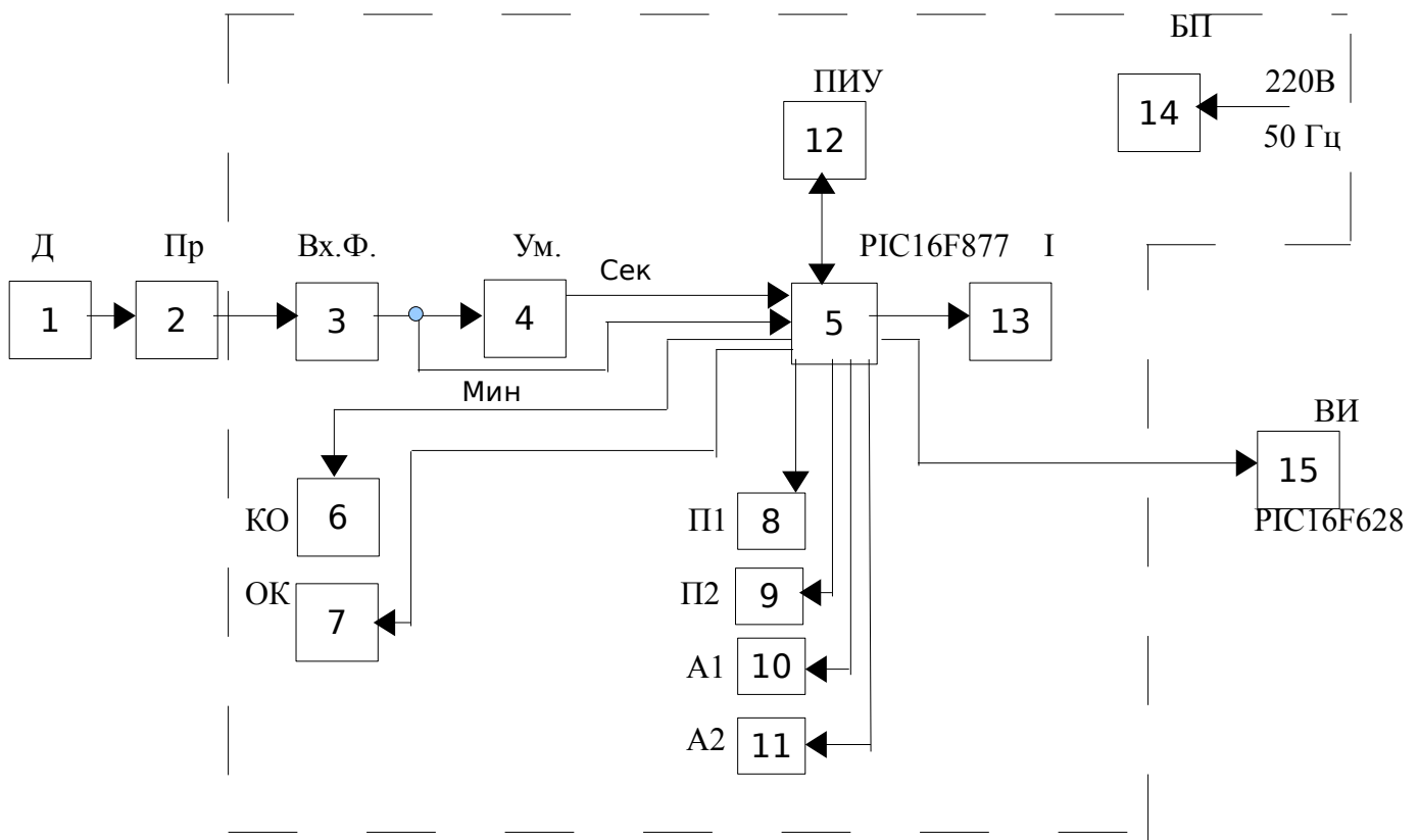
Рис. 1. Структурная схема тахометра ИП-114.
